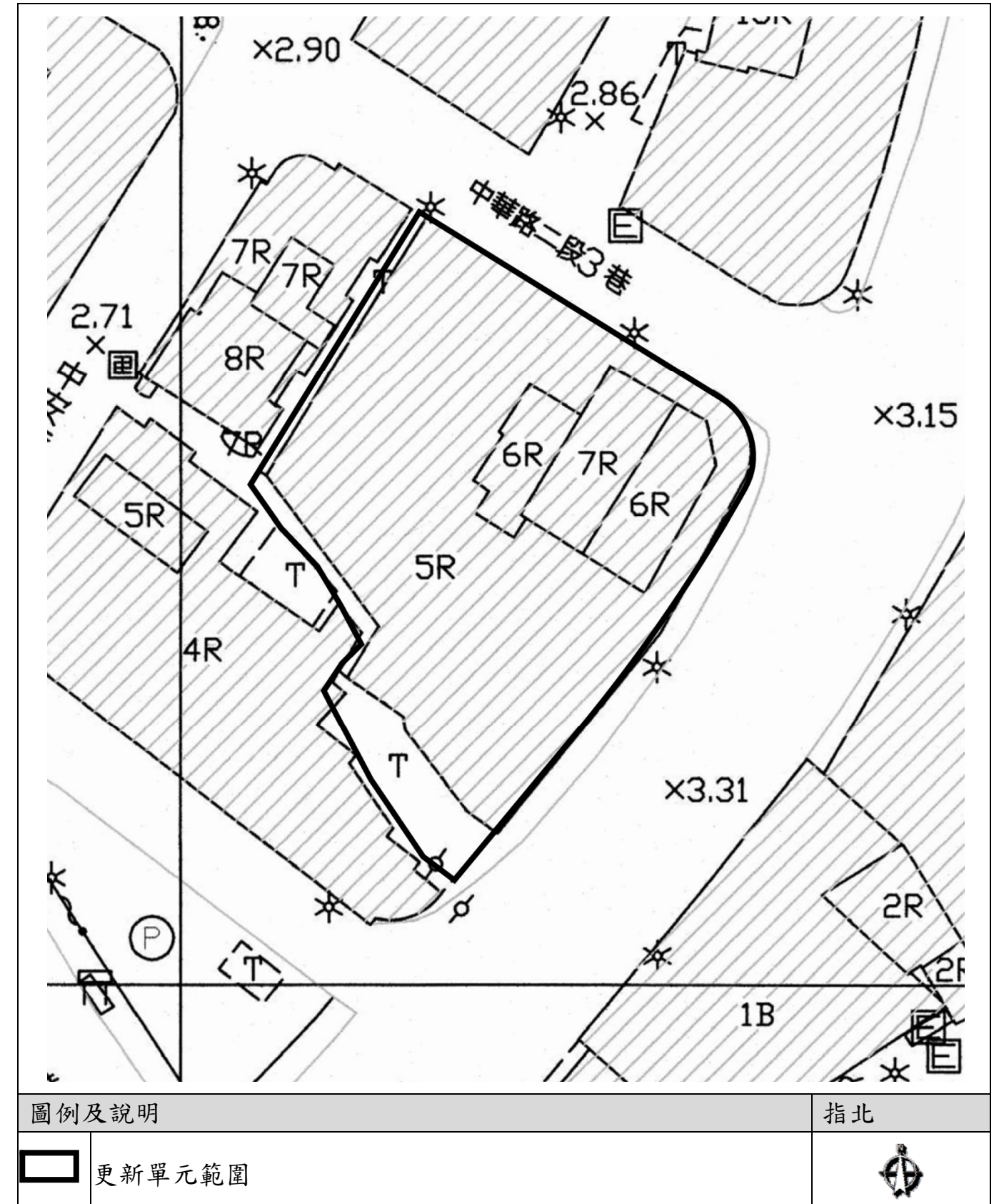
圖2-3 更新單元地形套繪圖 s:1/500
